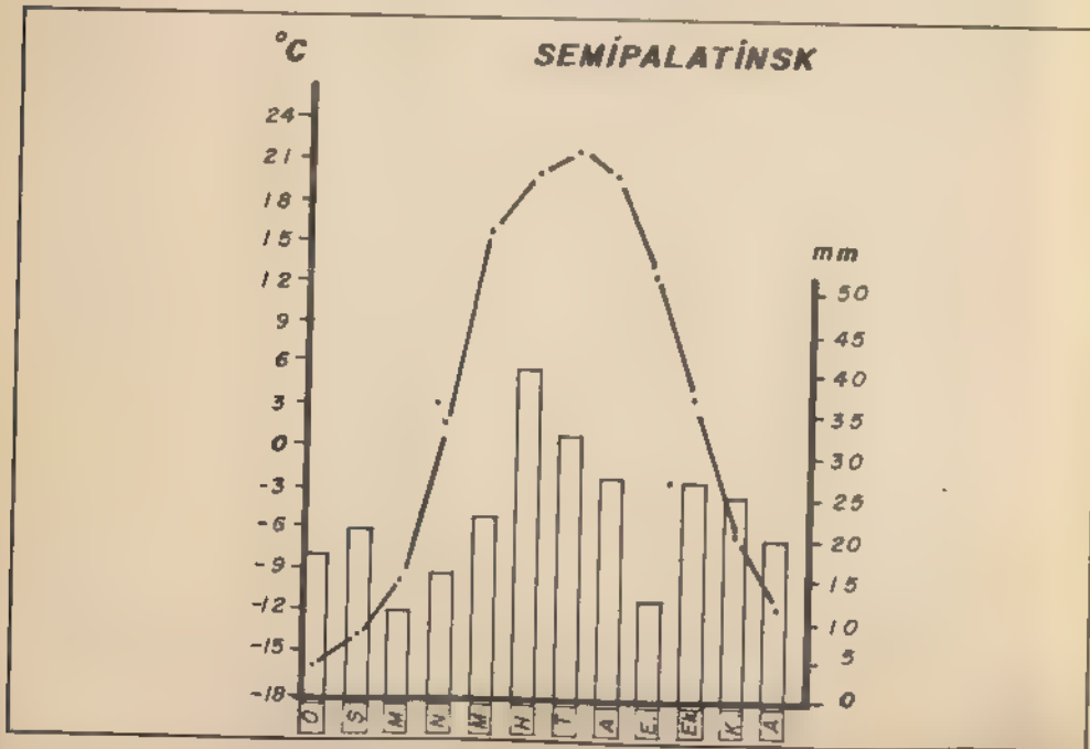
Şekil 5 - Semipalatinsk'in iklim diyagramı. Sıcaklık kesik çizgi ile, yağış sütunlarla gösterilmiştir
